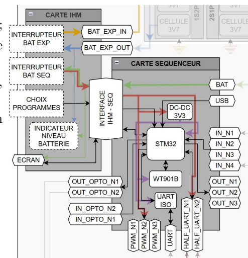
FIGURE 5.3 – Zoom sur le séquenceur et interface
