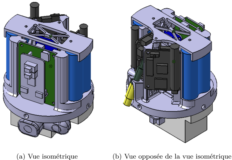
FIGURE 4.12 – Bloc électronique du premier étage sur CATIA
