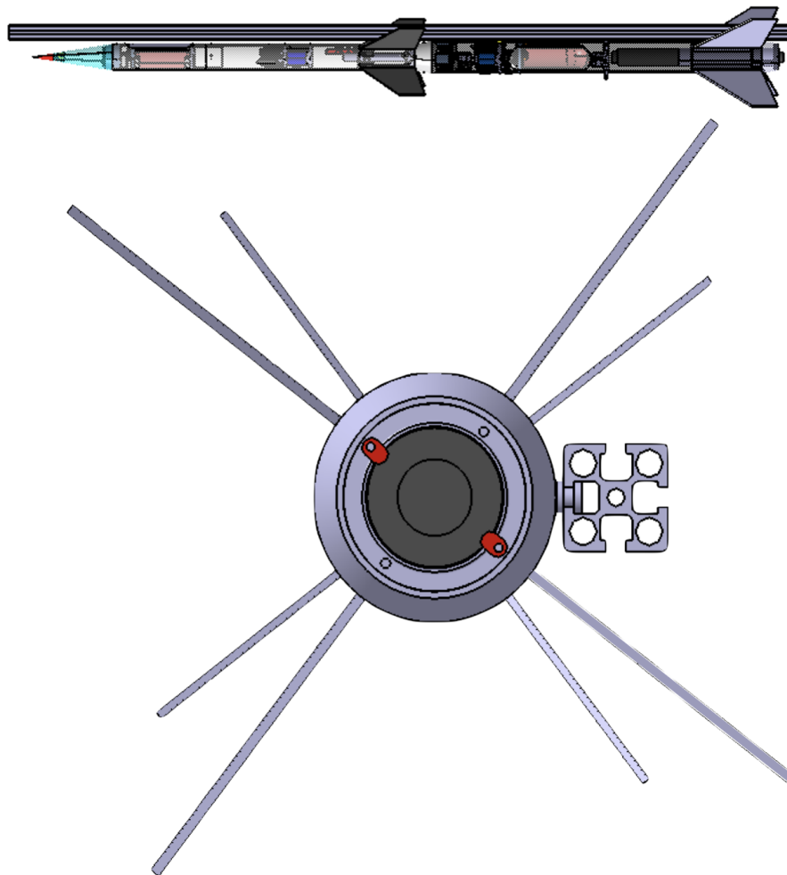
FIGURE 4.23 – Angles entre les ailerons proches de la rampe sur la configuration de mise en rampe
