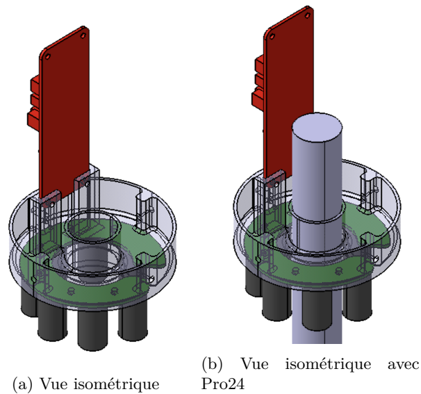
FIGURE 4.22 – Bloc électronique du second étage sur CATIA
