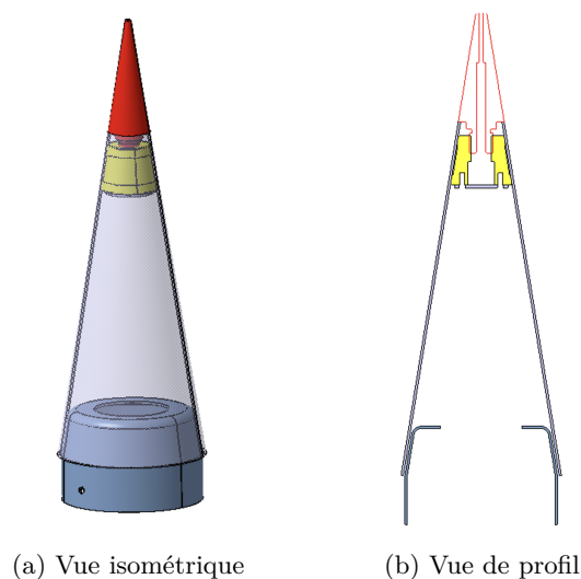
FIGURE 4.20 – Bloc électronique du second étage sur CATIA
