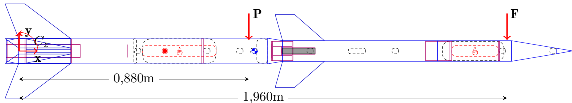
FIGURE 4.1 – Schéma de calcul du couple exercé au niveau de la base du premier étage
