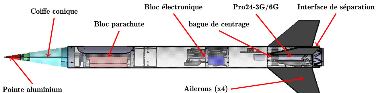
FIGURE 1.3 – Vue du second étage sur CATIA
